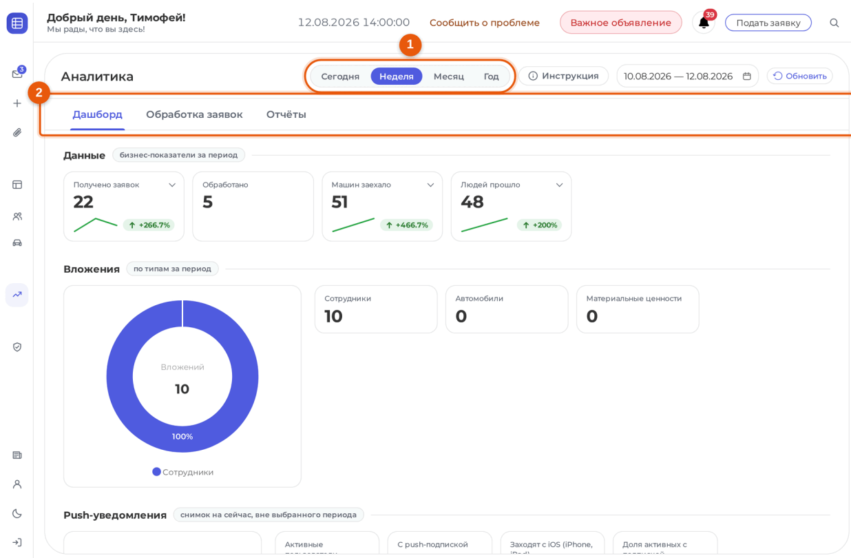
Рисунок 17.1 — Аналитика: дашборд
